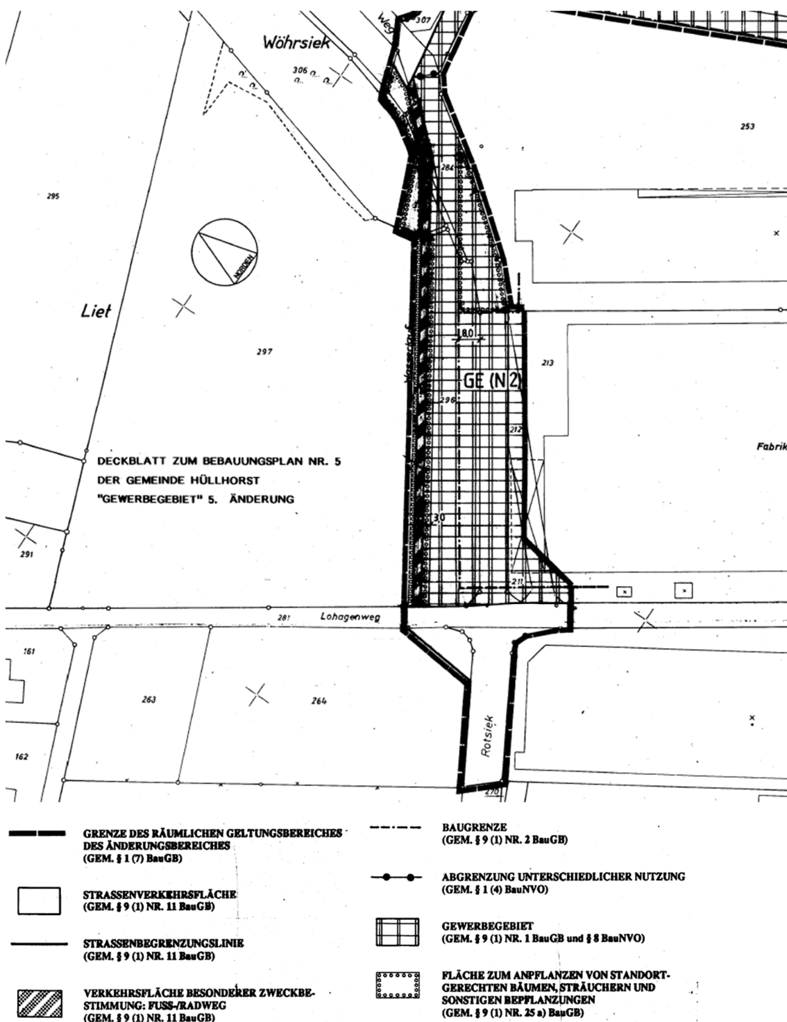
Abb. 4 Auszug der 5. Änderung des Bebauungsplans Nr. 5 „Gewerbegebiet“ der Gemeinde Hüllhorst (GEMEINDE HÜLLHORST 1998).
