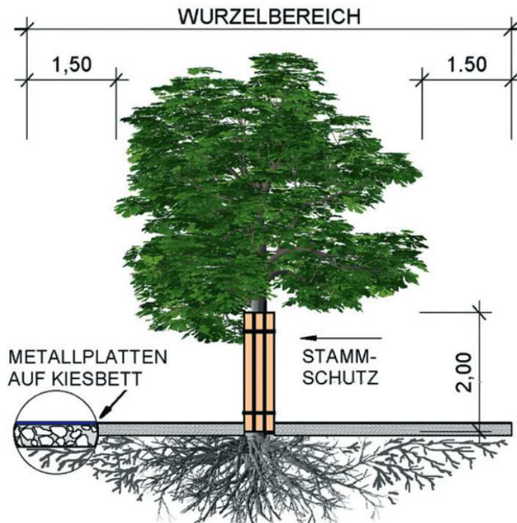
Abb. 6 Wurzel- und Stammschutzmaßnahmen nach RAS-LP4 bei zwingend notwendiger Befahrung des Wurzelbereichs (GALK 2014).
