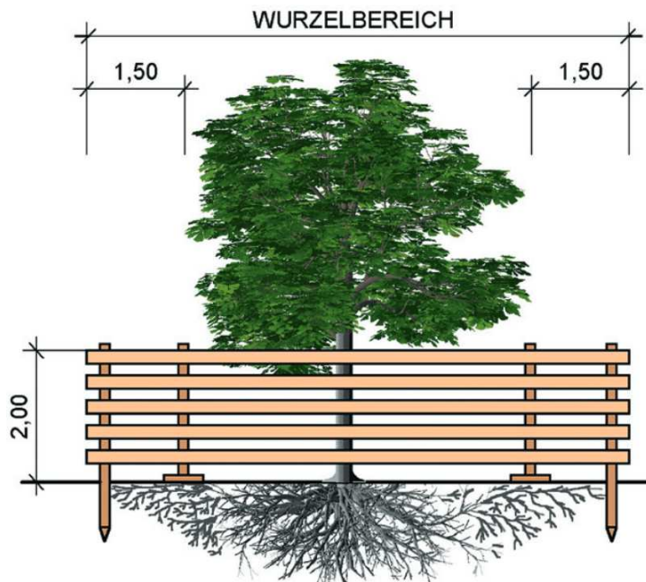
Abb. 5 Schutz des Wurzelbereichs durch ortsfesten Zaun nach RAS-LP4 (GALK 2014).
