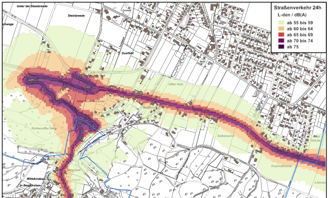
Karte 7: Isophonenkarte Tag L den L 876 und L 772, genordnet, ohne Maßstab (Auszug aus Anlage 8)
