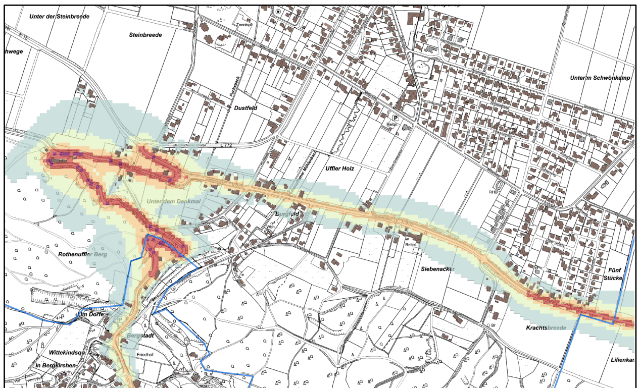
Karte 8: Isophonenkarte Nacht L_{night} L 876 und L 772, genordnet, ohne Maßstab (Auszug aus Anlage 9)
