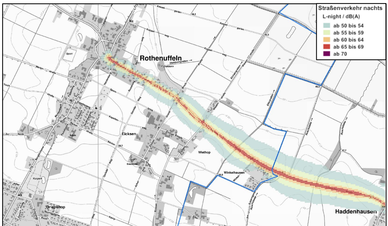
Karte 6: Isophonenkarte Nacht L_{night} B 65, genordnet, ohne Maßstab (Auszug aus Anlage 7)
