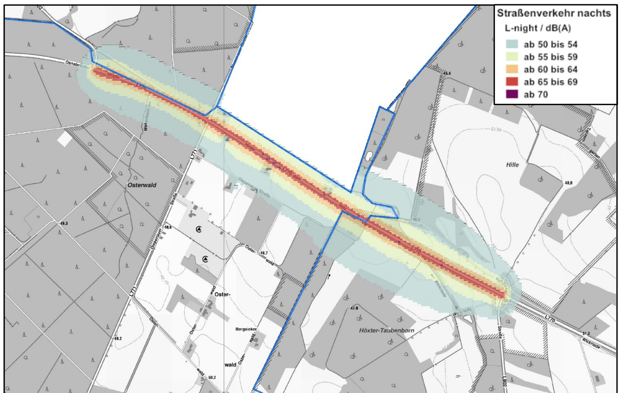
Karte 2: Isophonenkarte Nacht L_{night} L 770, genordnet, ohne Maßstab (Auszug aus Anlage 3)
