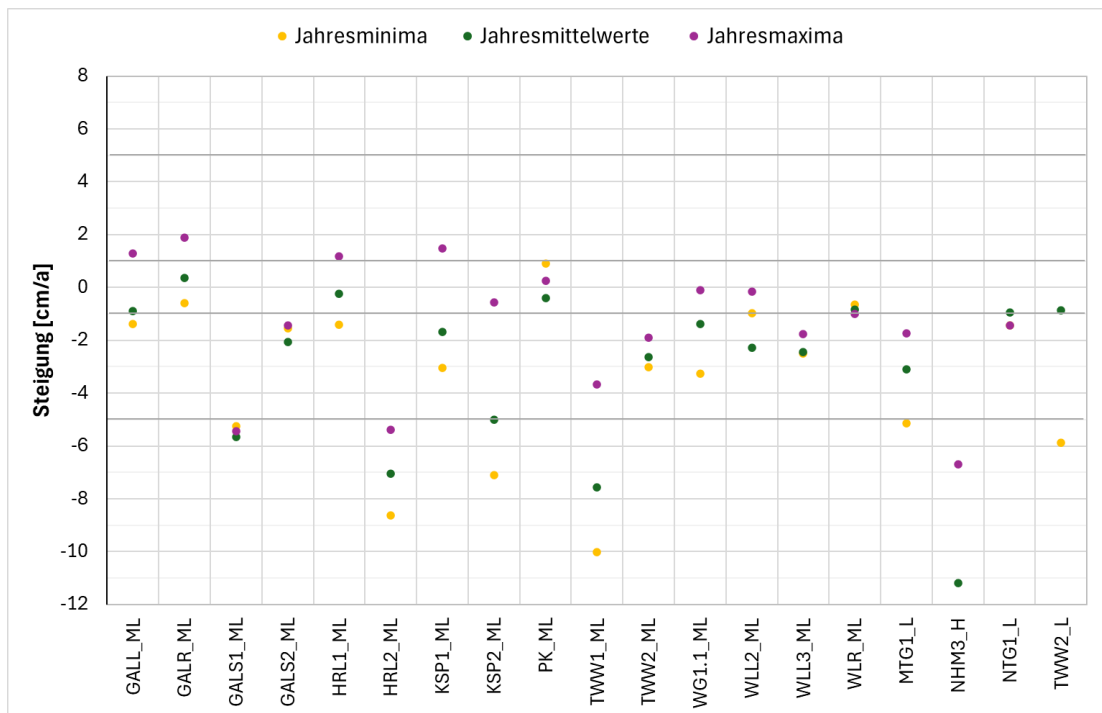
Abb. 2.8: Mittlere Steigung je Bilanzraum im Zeitraum 2011-2020
