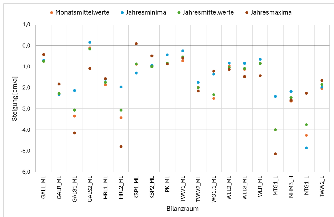
Abb. 2.3: Mittlere Steigung je Bilanzraum
