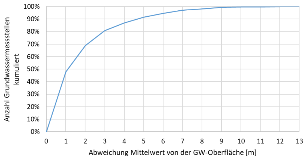
Abb. 1.2: Summenkurve der Abweichungen der Messstellen
