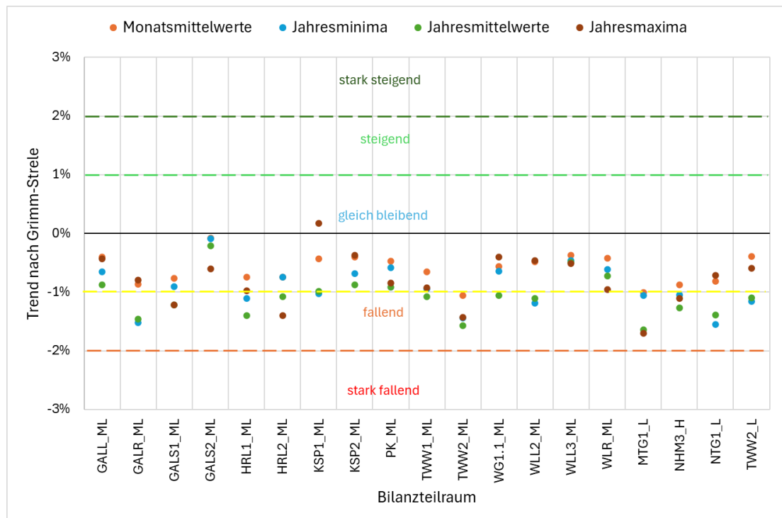
Abb. 2.4: Mittlere Trends nach Grimm-Strele je Bilanzraum
