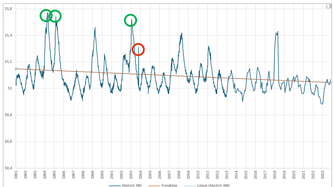
Abb. 2.2: Beispielganglinie: grüne Kreise: hohe Abweichungen von der Regressionsgeraden, die aber wahrscheinlich klimatisch bedingt sind und somit keine Ausreißer sind; roter Kreis: vermuteter Ausreißer, der aber gemäß statistischer Auswertung definitionsgemäß kein Ausreißer ist.
