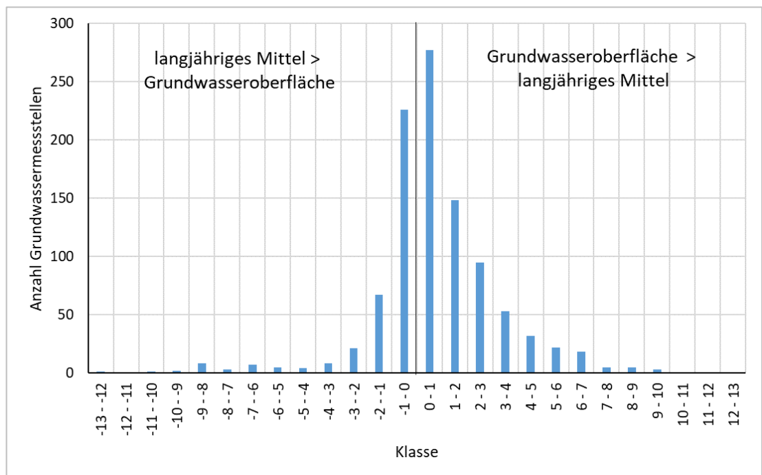
Abb. 1.1: Verteilung der absoluten Abweichungen der langjährigen Mittelwerte von der Grundwasseroberfläche für mittlere Verhältnisse
