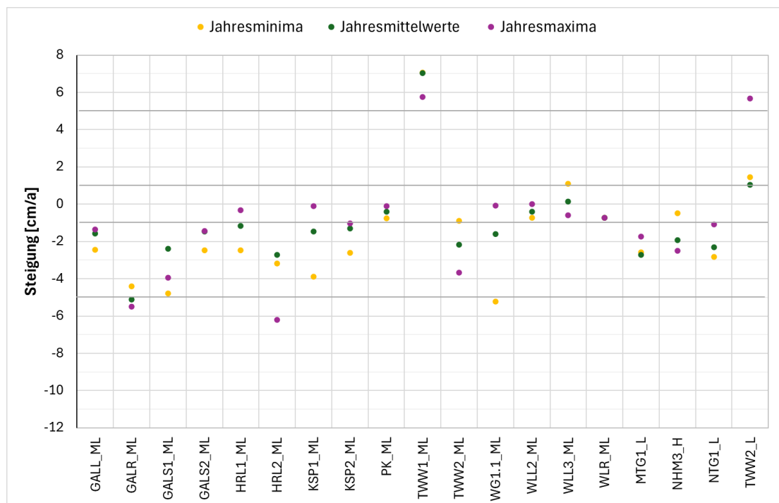
Abb. 2.7: Mittlere Steigung je Bilanzraum im Zeitraum 2001-2010
