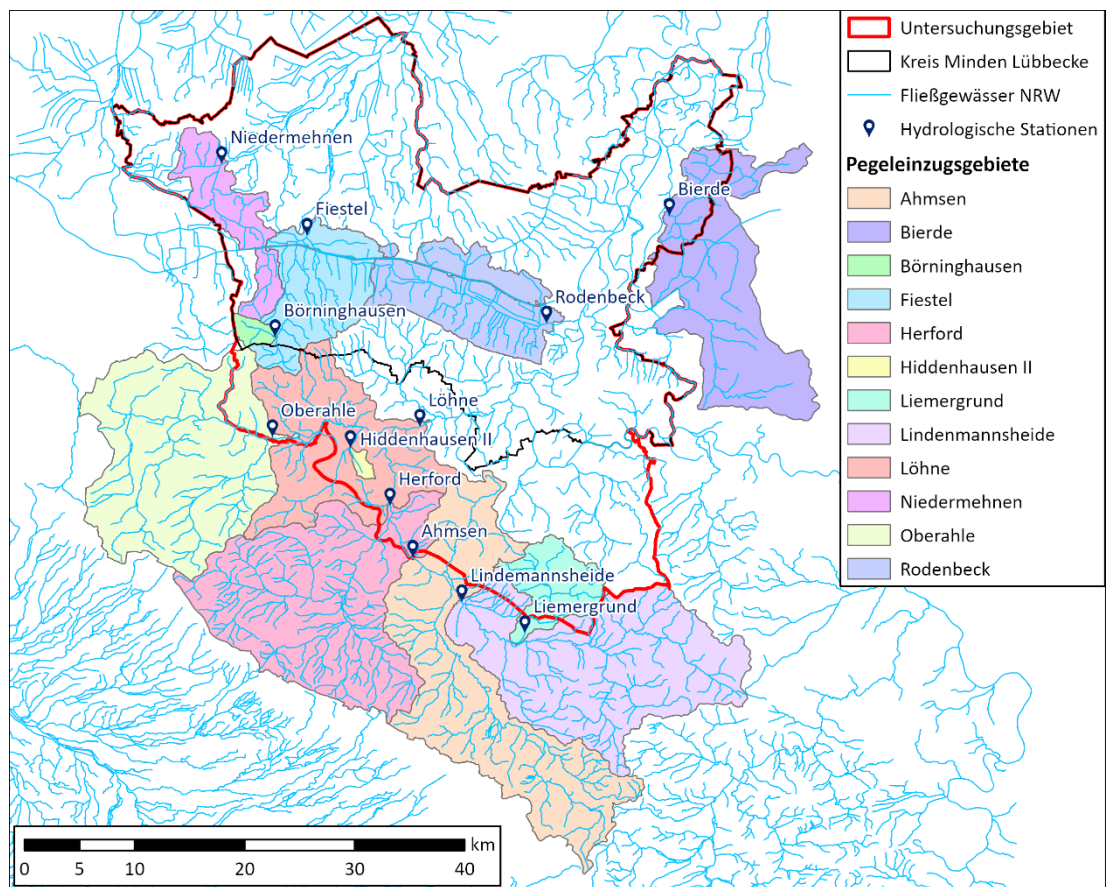
Abb. 3.1: Oberflächenwasserpegel mit Einzugsgebiet im Projektgebiet
