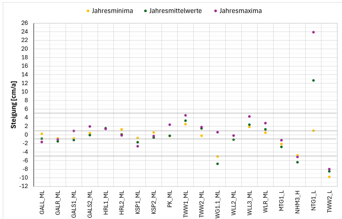
Abb. 2.6: Mittlere Steigung je Bilanzraum im Zeitraum 1991-2000
