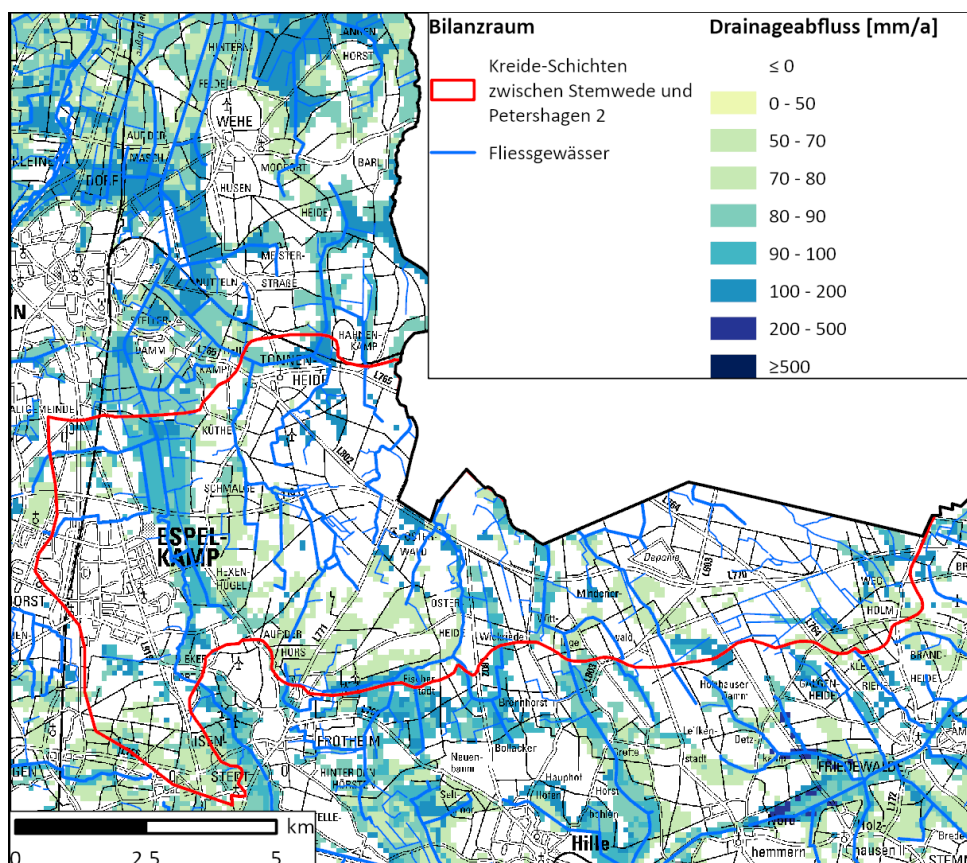
Abb. 19.1: Bilanzraum Kreide-Schichten zwischen Stemwede und Petershagen 2 und dessen Drainageflächen
