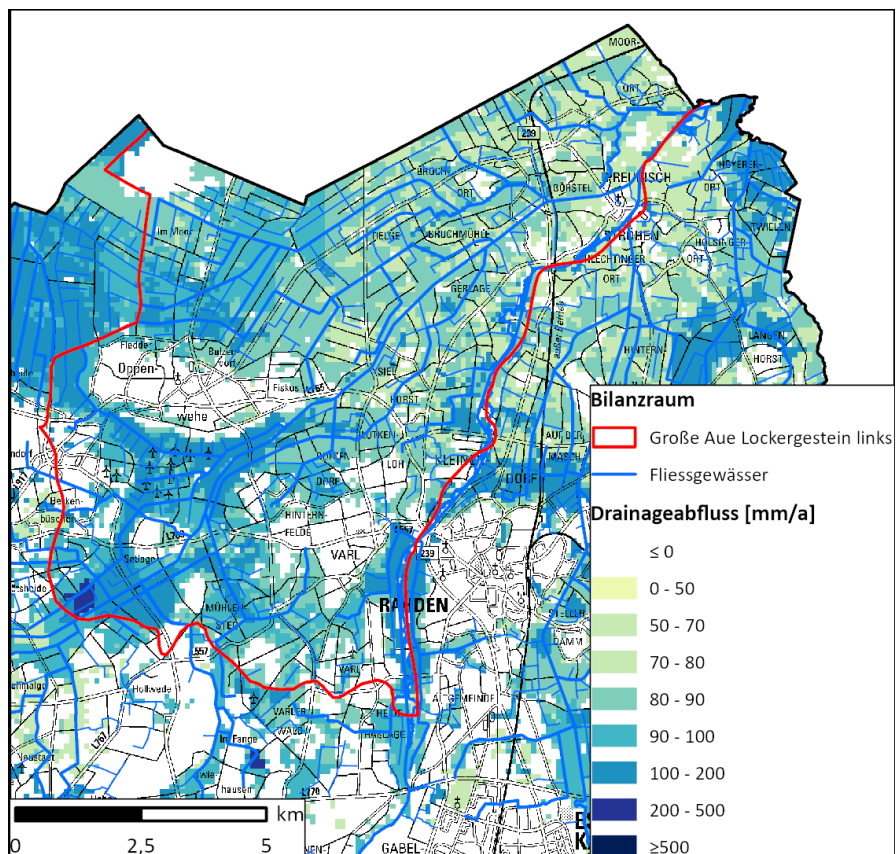
Abb. 16.1: Bilanzraum Große Aue Lockergestein links und dessen Drainageflächen
