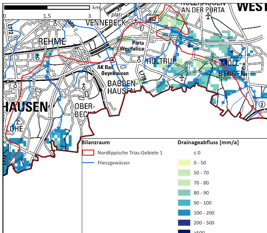
Abb. 15.1: Bilanzraum Nordlippische Trias-Gebiete und dessen Drainageflächen
