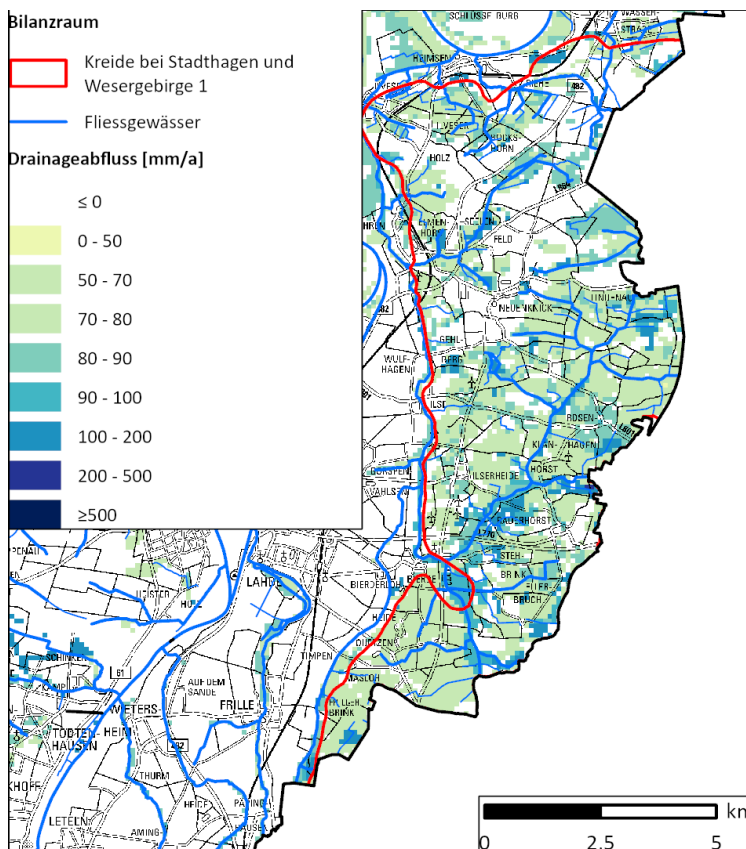
Abb. 6.1: Bilanzraum Kreide bei Stadthagen und Wesergebirge 1 und dessen Drainageflächen
