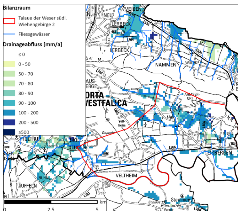
Abb. 10.1: Bilanzraum Talaue der Weser südl. Wiehengebirge 2 und dessen Drainageflächen
