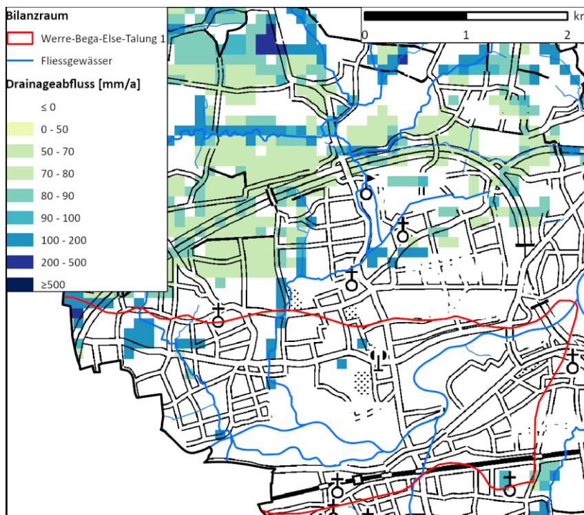
Abb. 13.1: Bilanzraum Werre-Bega-Else-Talung und dessen Drainageflächen
