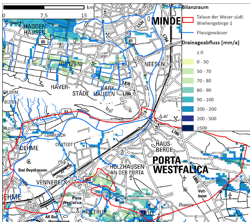
Abb. 9.1: Bilanzraum Talaue der Weser südl. Wiehengebirge 1 und dessen Drainageflächen
