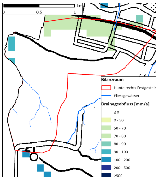
Abb. 24.1: Bilanzraum Hunte rechts Festgestein und dessen Drainageflächen
