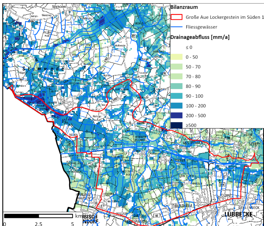
Abb. 20.1: Bilanzraum Große Aue Lockergestein im Süden 1 und dessen Drainageflächen
