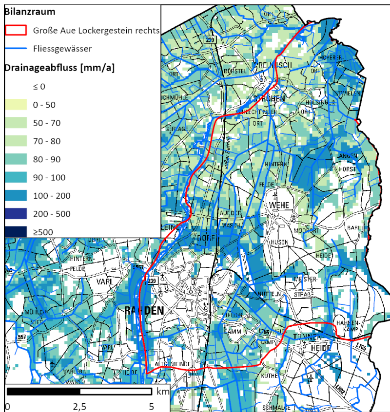
Abb. 17.1: Bilanzraum Große Aue Lockergestein rechts und dessen Drainageflächen
