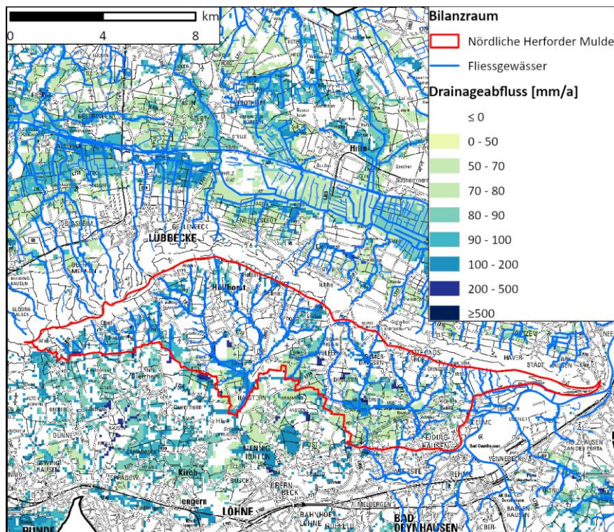
Abb. 12.1: Bilanzraum Nördliche Herforder Mulde und dessen Drainageflächen
