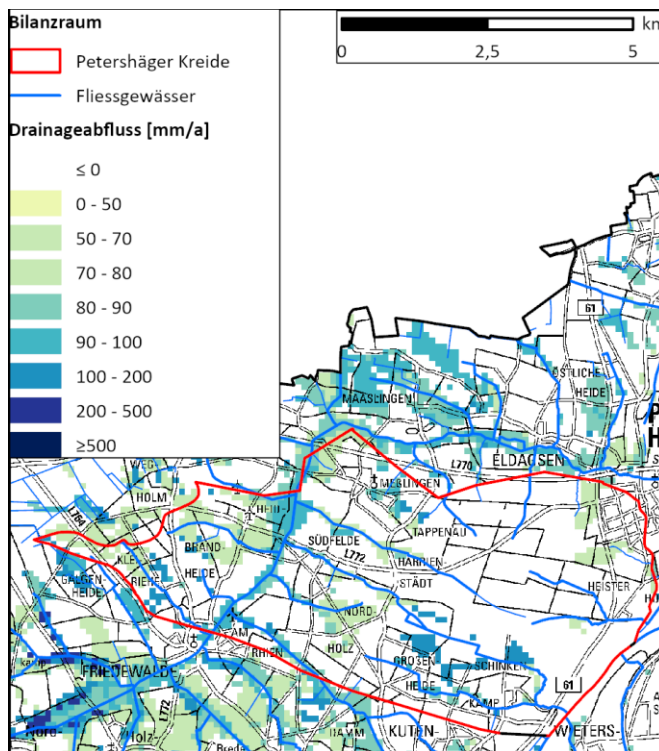
Abb. 5.1: Bilanzraum Petershäger Kreide und dessen Drainageflächen
