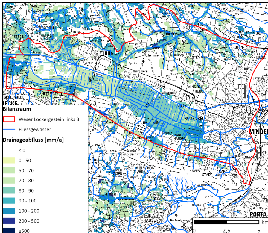
Abb. 4.1: Bilanzraum Weser Lockergestein links 3 und dessen Drainageflächen
