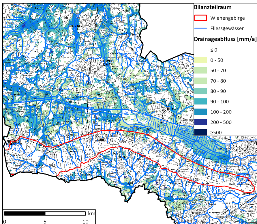
Abb. 11.1: Bilanzraum Wiehengebirge und dessen Drainageflächen
