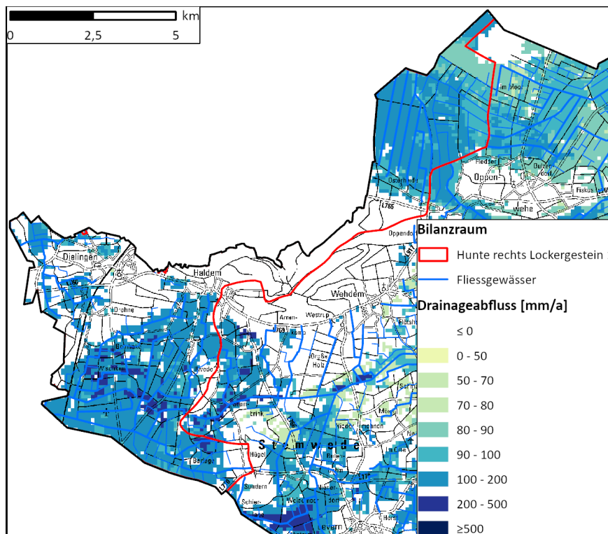
Abb. 22.1: Bilanzraum Hunte rechts Lockergestein 1 und dessen Drainageflächen
