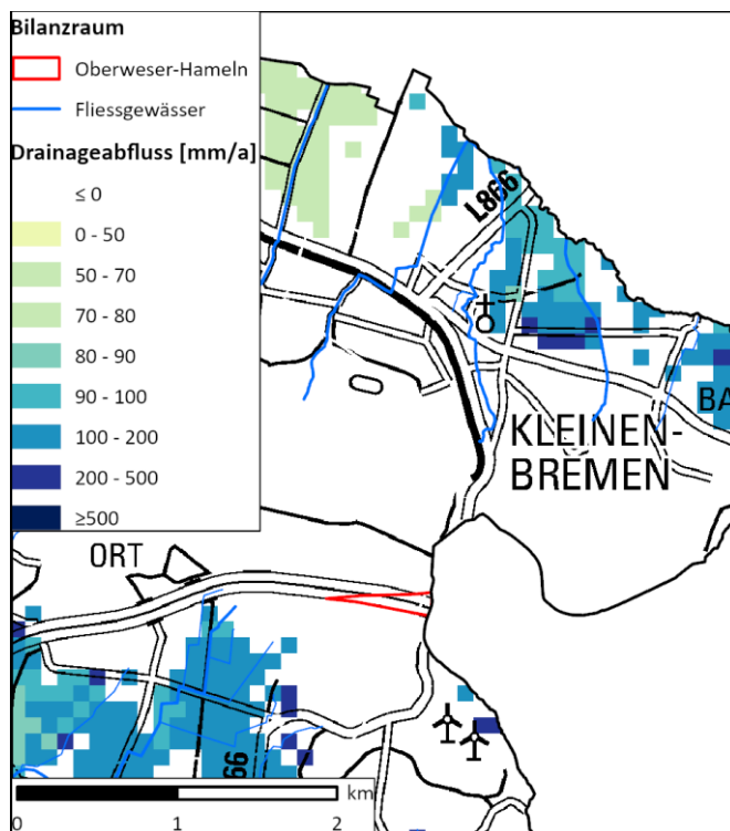
Abb. 8.1: Bilanzraum Oberweser-Hameln und dessen Drainageflächen
