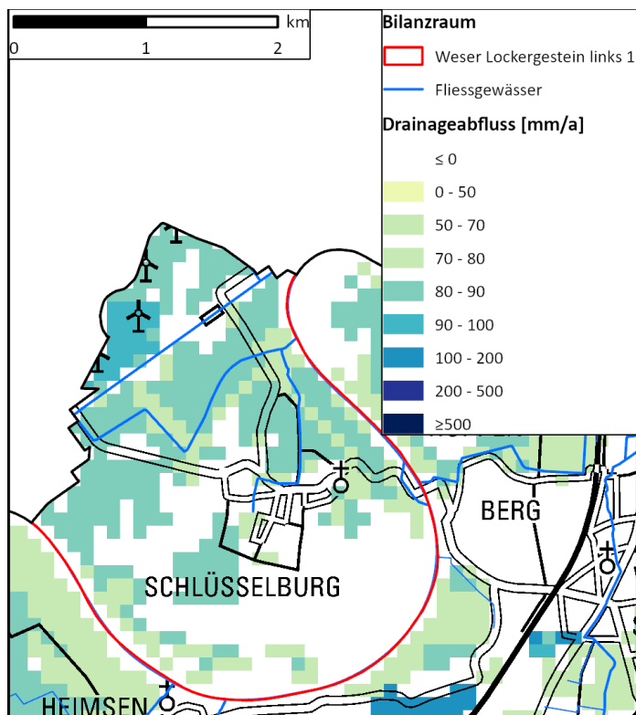
Abb. 2.1: Bilanzraum Weser Lockergestein links 1 und dessen Drainageflächen
