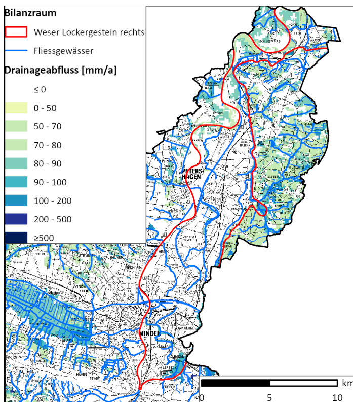
Abb. 1.1: Bilanzraum Weser Lockergestein rechts und dessen Drainageflächen
