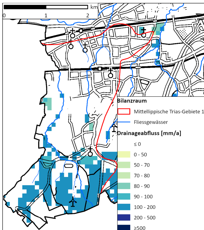
Abb. 14.1: Bilanzraum Mittellippische Trias-Gebiete und dessen Drainageflächen
