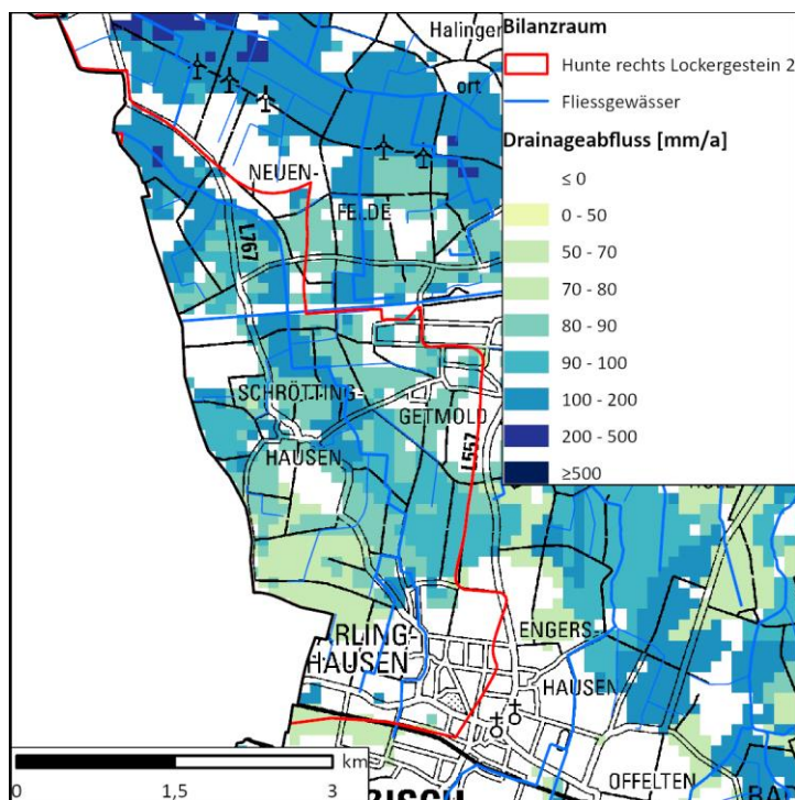
Abb. 23.1: Bilanzraum Hunte rechts Lockergestein 2 und dessen Drainageflächen
