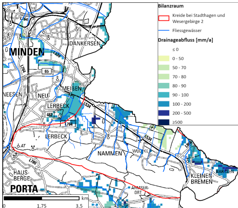
Abb. 7.1: Bilanzraum Kreide bei Stadthagen und Wesergebirge 2 und dessen Drainageflächen
