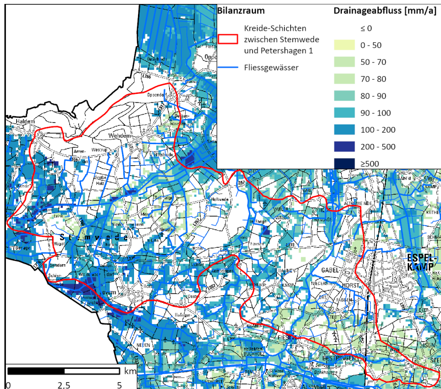
Abb. 18.1: Bilanzraum Kreide-Schichten zwischen Stemwede und Petershagen 1 und dessen Drainageflächen
