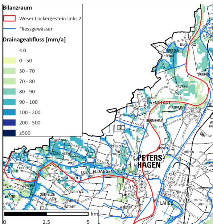
Abb. 3.1: Bilanzraum Weser Lockergestein links 2 und dessen Drainageflächen
