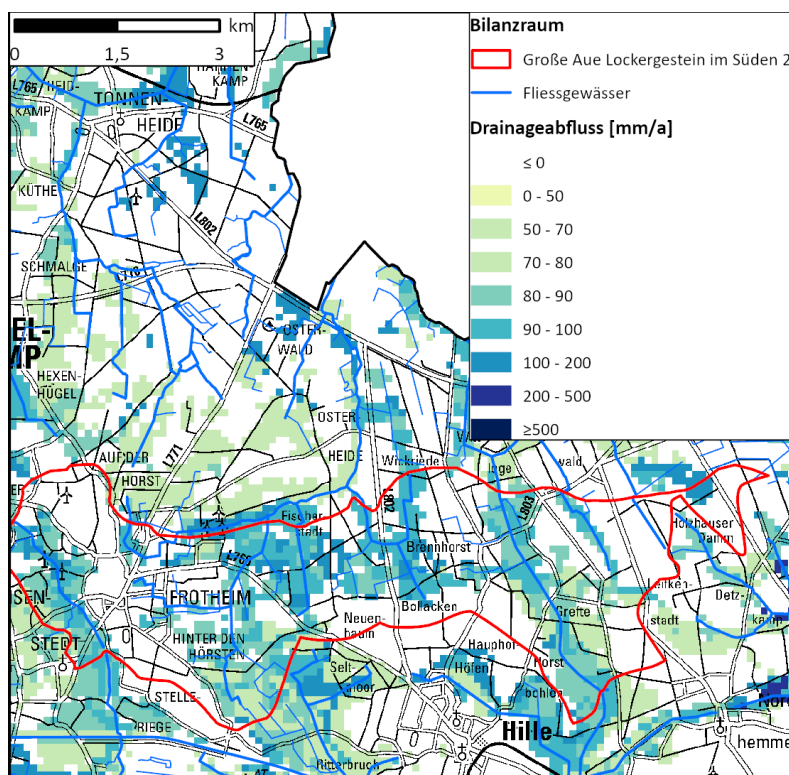
Abb. 21.1: Bilanzraum Große Aue Lockergestein im Süden 2 und dessen Drainageflächen
