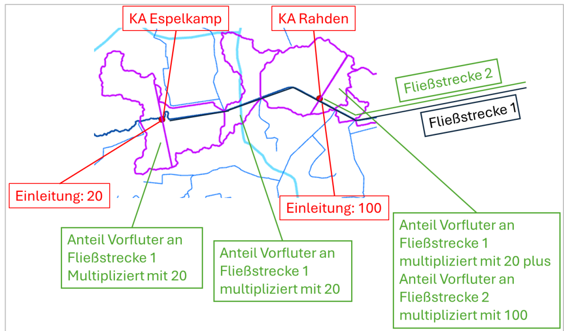
Abb. 6.15: Prinzipskizze Variante 2 der Berücksichtigung von Kläranlageneinleitungen als Bilanzgröße
