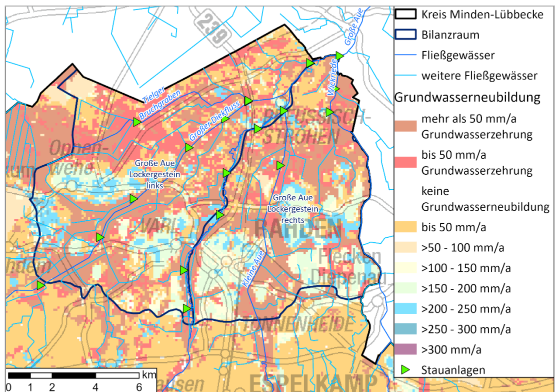
Abb. 6.7: Bilanzräume Große Aue Lockergestein links und rechts mit relevanten Fließgewässern und Grundwasserneubildung im Istzustand.
