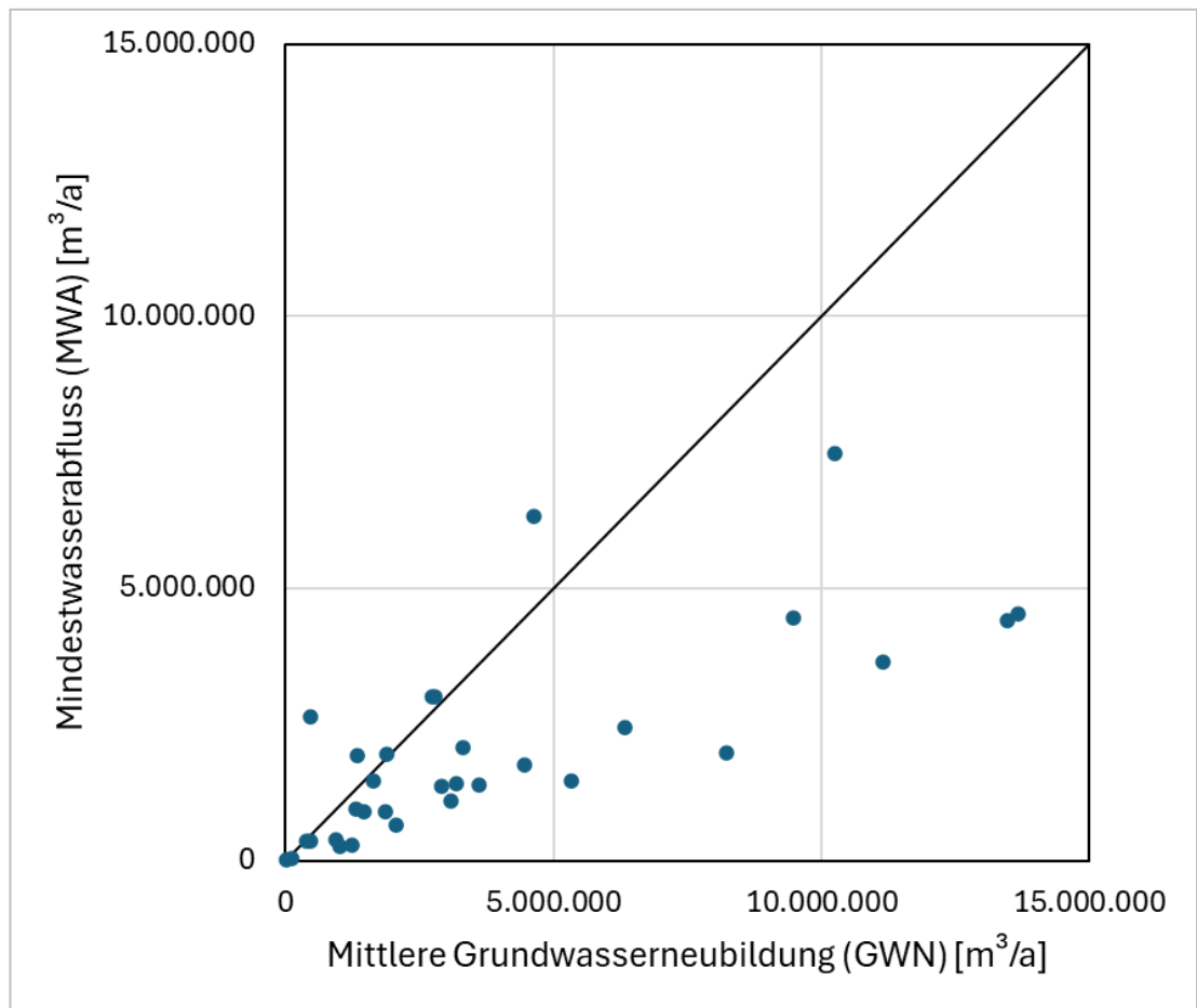
Abb. 7.3: Verhältnis der mittleren Grundwasserneubildung zum Mindestwasserabfluss
