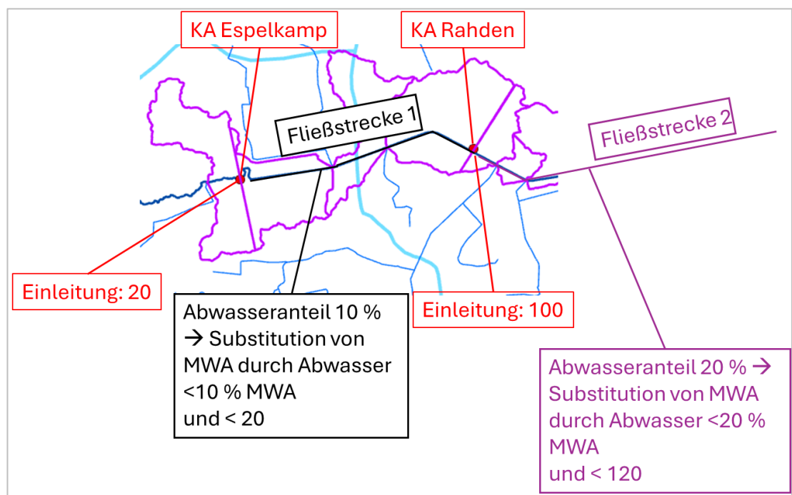
Abb. 6.17: Prinzipskizze Variante 4 der Berücksichtigung von Kläranlageneinleitungen als Bilanzgröße
