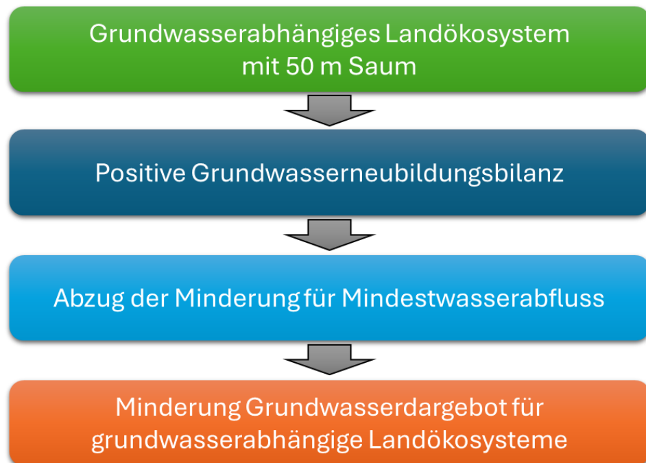
Abb. 7.8: Reduzierung des Grundwasserdargebots zur Sicherung grundwasserabhängiger Landökosysteme
