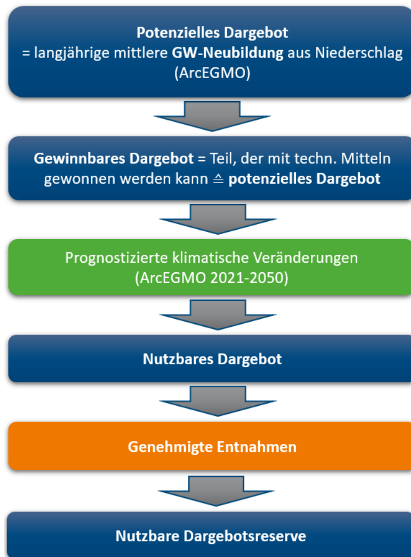
Abb. 4.5: Ablaufschema zur Ermittlung der nutzbaren Grundwasserdargebotsreserve im Land Sachsen
