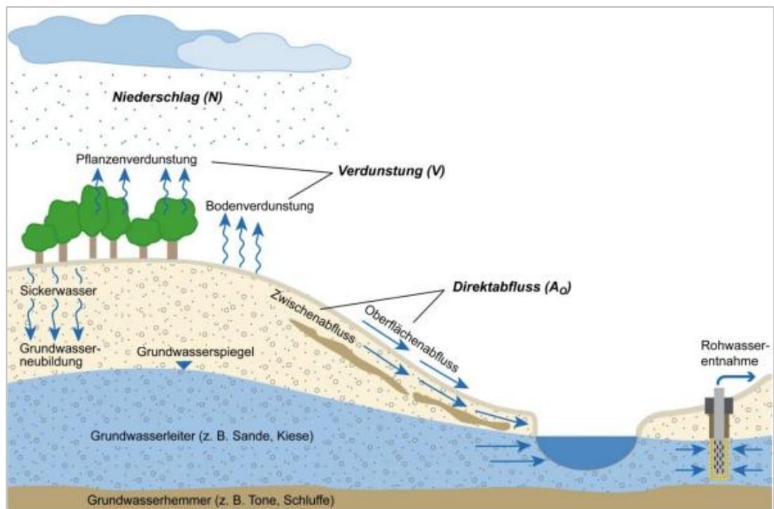
Abb. 3.1: Darstellung der Grundwasserhaushaltskomponenten (verändert nach BLOMENHOFER et al, 2012)
