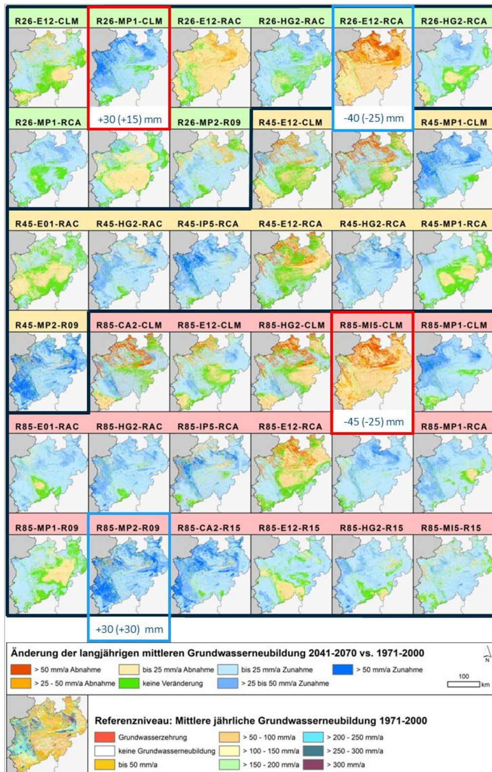
Abb. 6.6: Räumlich verteilte Änderungssignale der projizierten Grundwasserneubildung (2041-2070 vs. 1971-2000). Das RCP2.6-Teilensembel ist grün hinterlegt und das RCP8.5-Teilensembel ist rot hinterlegt. Rot umrandet: die gewählten Projektionspfade zur Begrenzung der Bandbreite; blau umrandet: Projektionspfade gegenteiliger Änderungssignale. Aus LANUV, 2021
