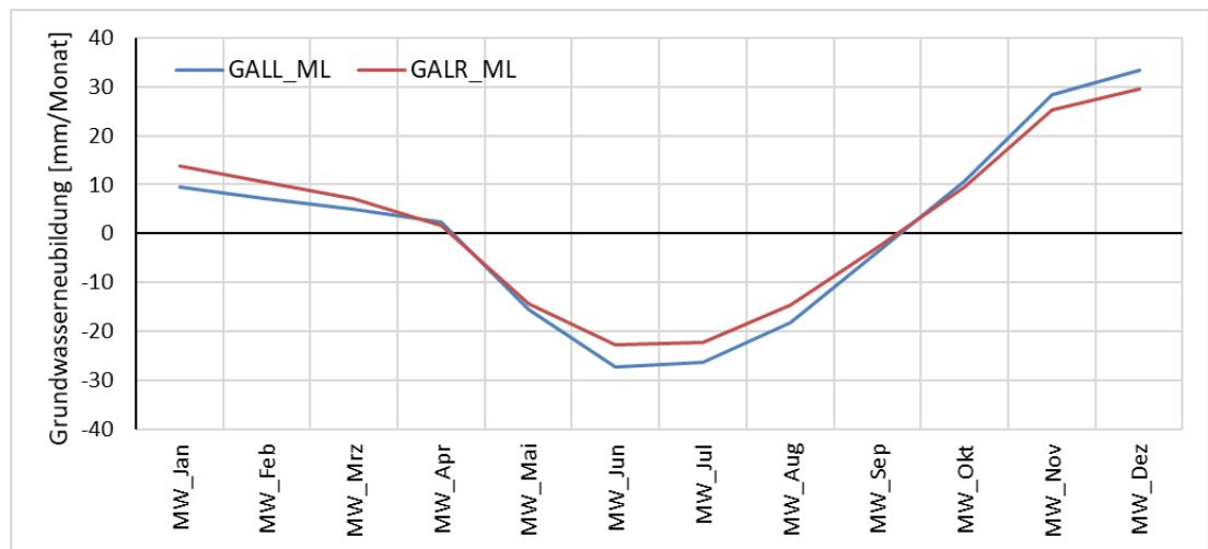
Abb. 6.8: Zeitreihe der langjährigen Monatsmittelwerte der Grundwasserneubildung in den Bilanzräumen Große Aue Lockergestein links und rechts
