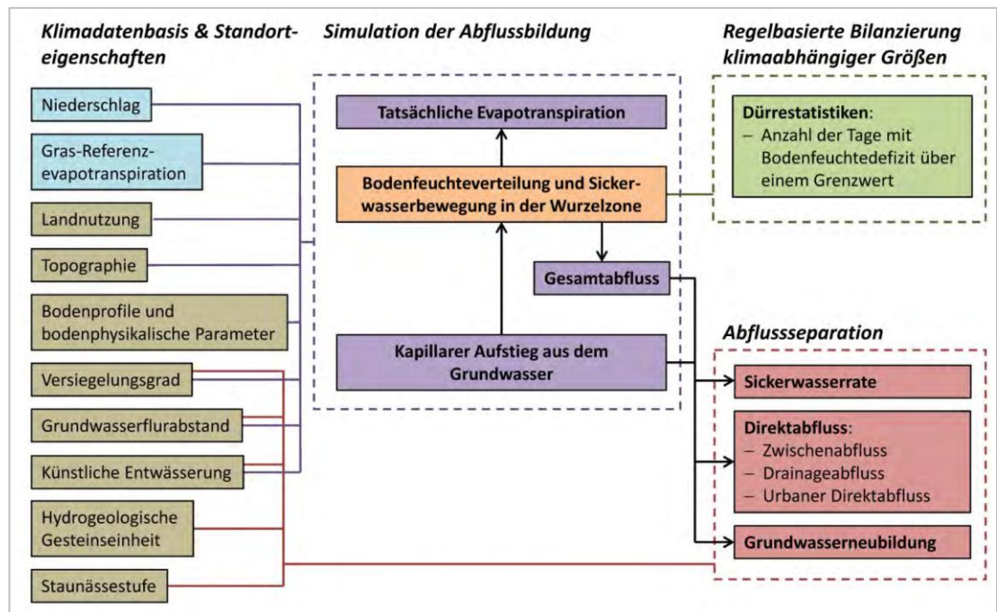
Abb. 6.1: Modellkonzept des Wasserhaushaltsmodells mGROWA in der Implementierung für Nordrhein-Westfalen (Quelle: LANUV-Fachbericht 110, Teil IIa, S. 14)
