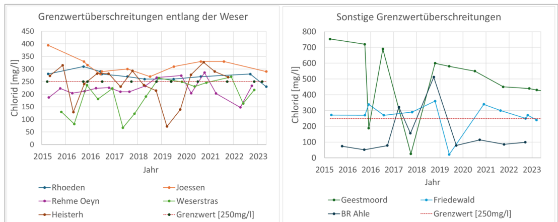
Abb. 7.10: Chloridkonzentrationsganglinien über die letzten 10 Jahre
