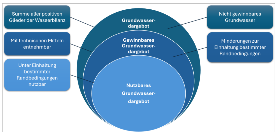
Abb. 7.1: Grundwasserdargebotsarten nach DIN 4049-3 (1994)
