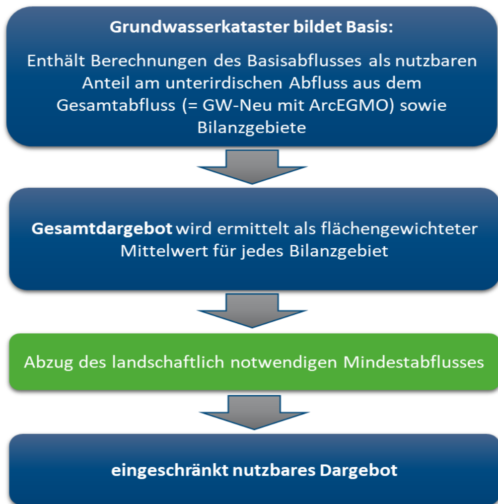
Abb. 4.6: Ablaufschema zur Ermittlung des eingeschränkt nutzbaren Grundwasserdargebots im Land Sachsen-Anhalt
