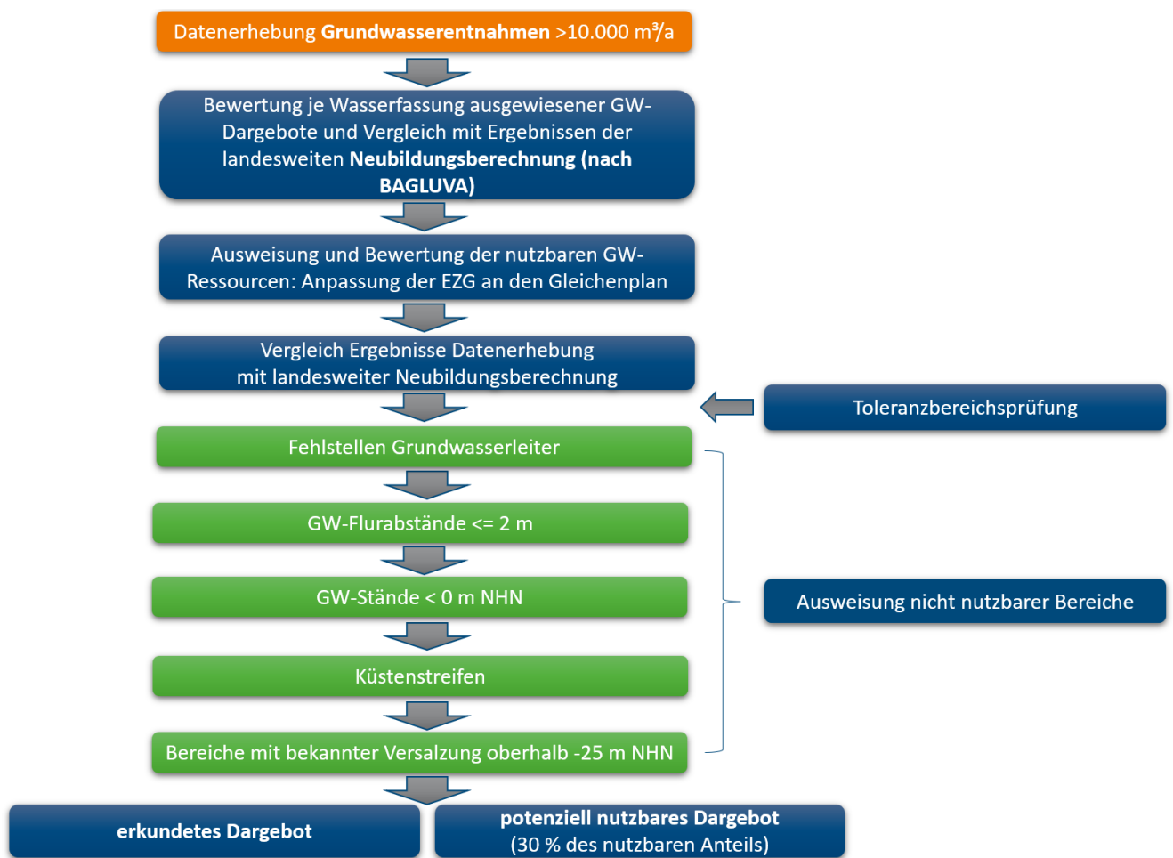
Abb. 4.2: Fließschema der Ermittlung des verfügbaren Grundwasserdargebotes im Land Mecklenburg-Vorpommern
