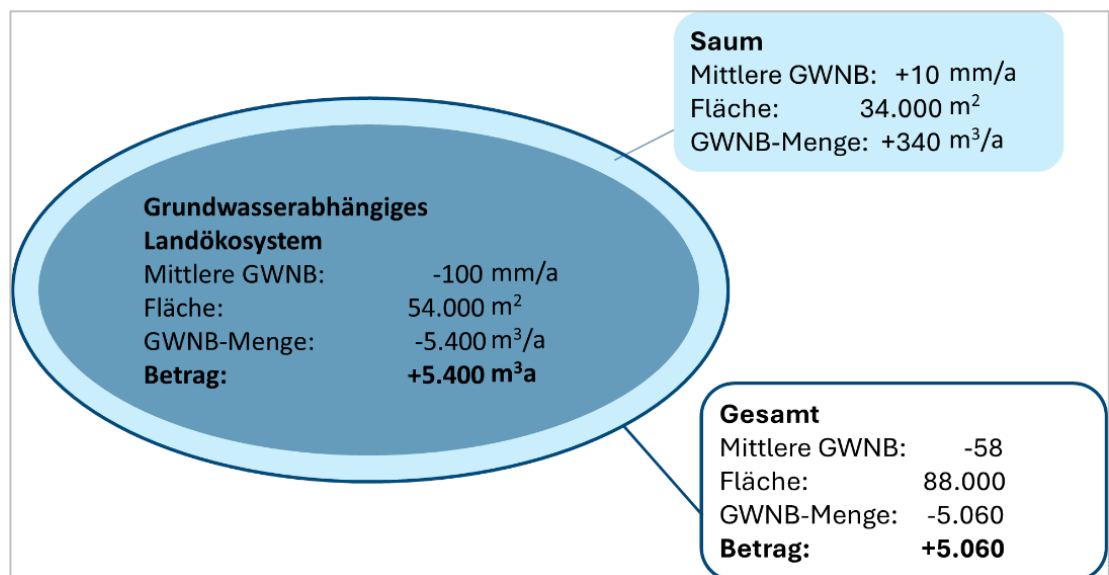
Abb. 7.5 Schematische Darstellung der Verringerung der Grundwasserneubildungsmenge bei Verwendung eines Saumes in der Bewertung
