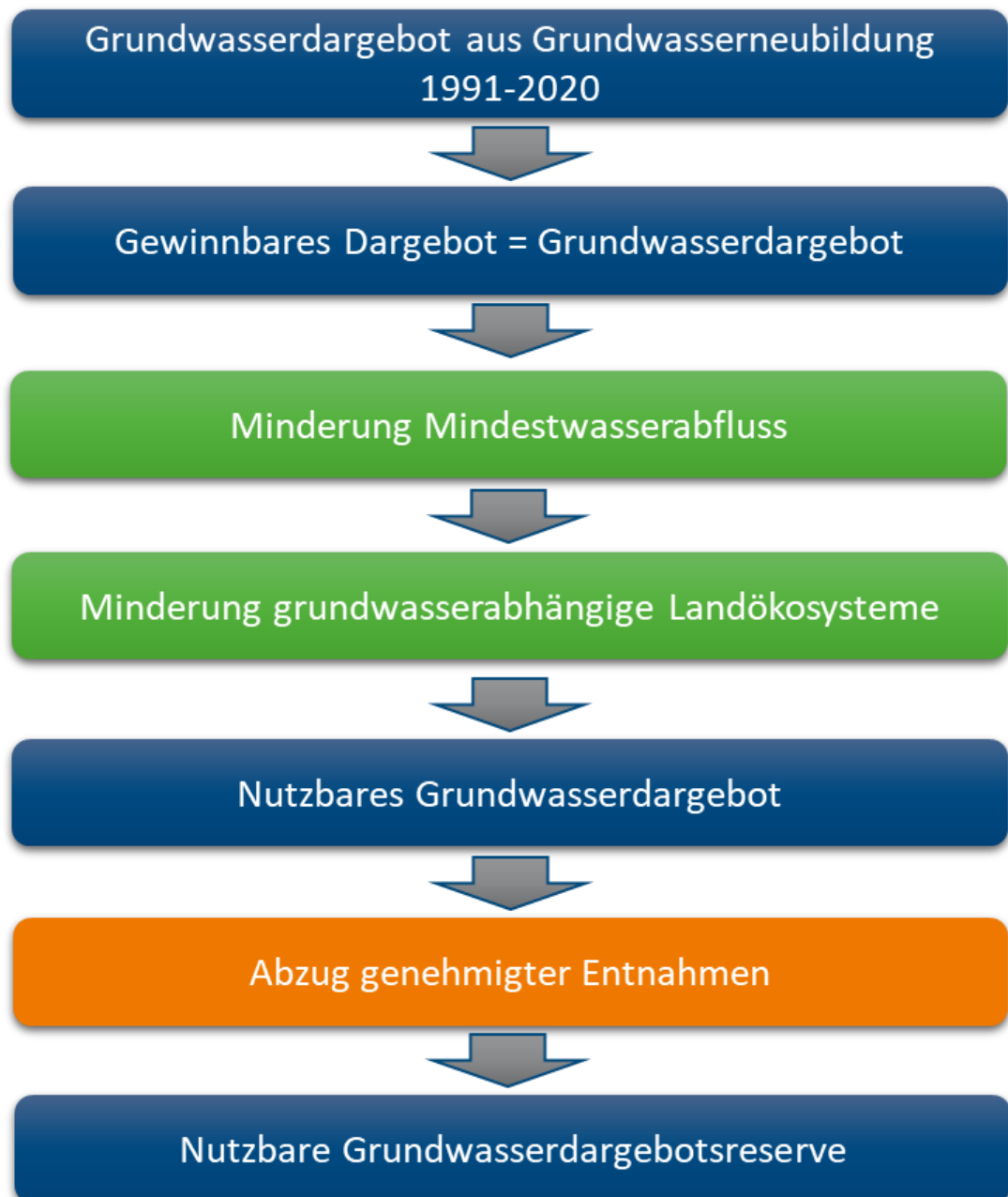
Abb. 9.1: Fließschema der Ermittlung des nutzbare Grundwasserdargebots entsprechend dem aufgestellten Konzept
