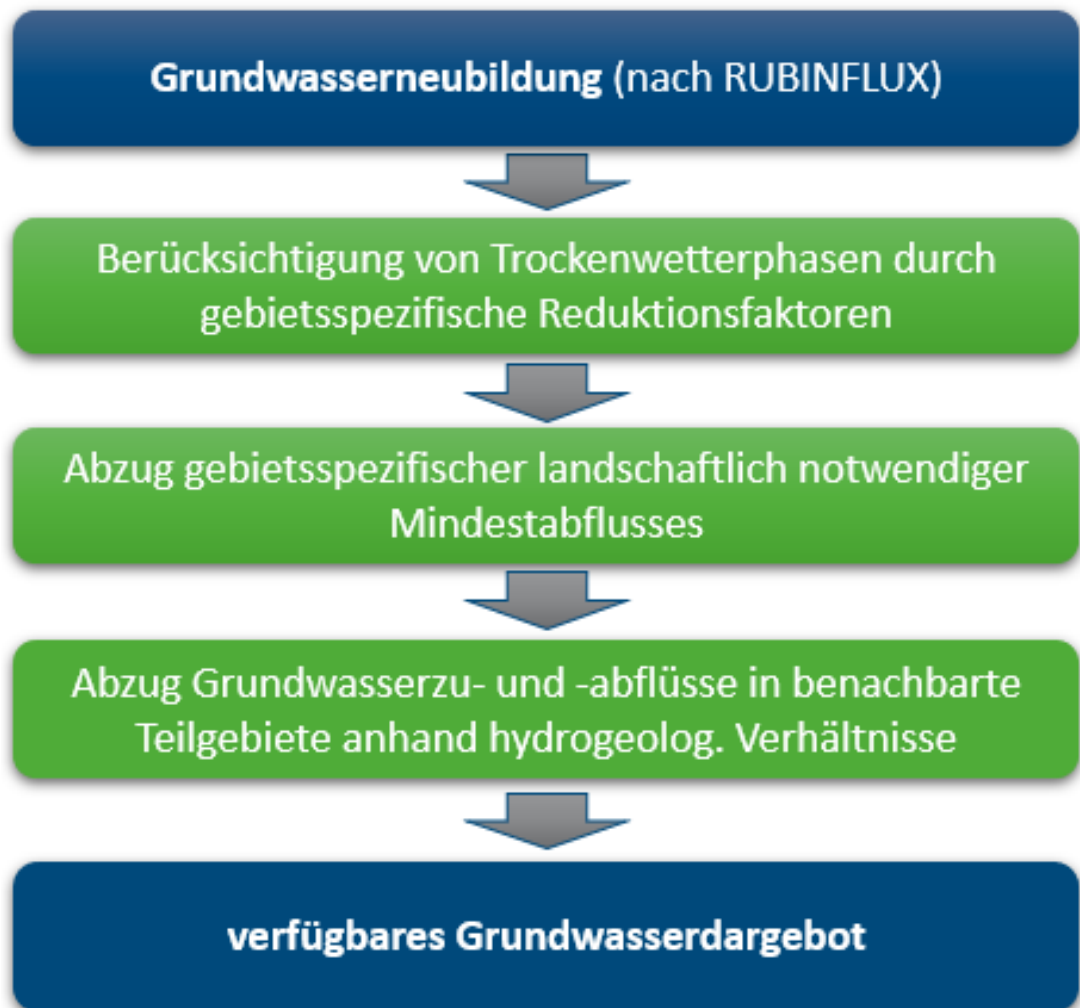
Abb. 4.7: Ablaufschema zur Ermittlung des verfügbaren Grundwasserdargebots im Land Thüringen
