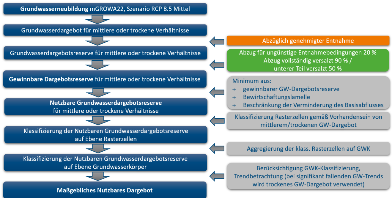
Abb. 4.4: Ablaufschema zur Ermittlung des maßgeblichen nutzbaren Grundwasserdargebots im Land Niedersachsen gemäß aktuellem Mengenerlass
