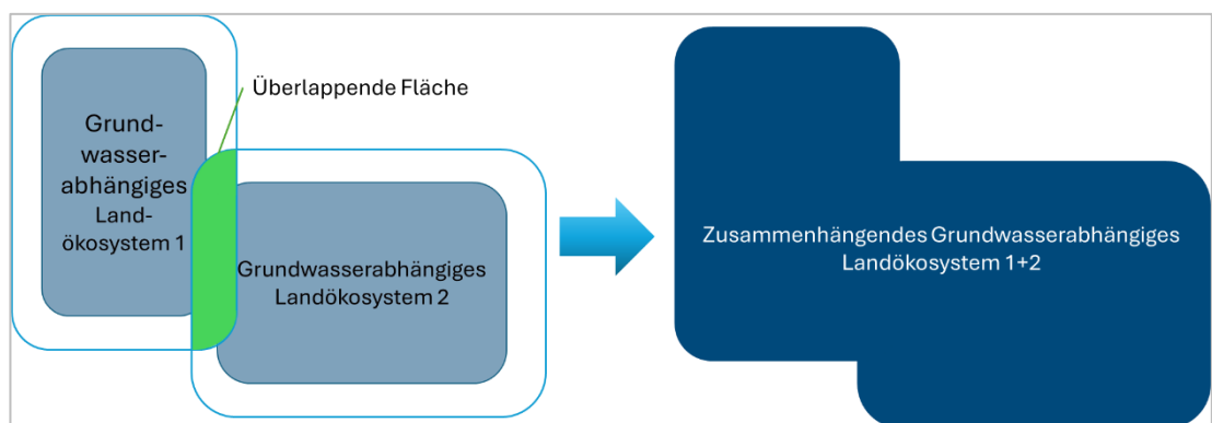
Abb. 7.7: Schematische Darstellung der Auswertung nahegelegener grundwasserabhängiger Landökosysteme
