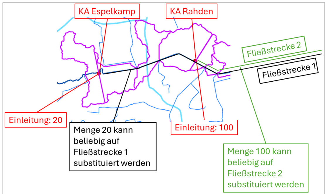
Abb. 6.16: Prinzipskizze Variante 3 der Berücksichtigung von Kläranlageneinleitungen als Bilanzgröße
