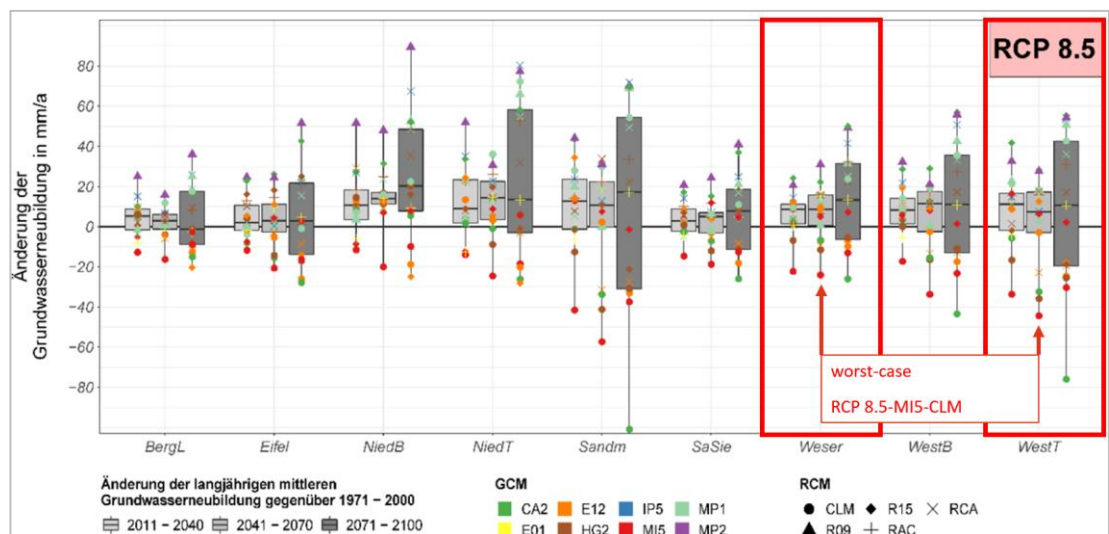
Abb. 6.5: Boxplots der Änderungssignale der langjährigen mittleren Grundwasserneubildung im RCP Teilensembel RCP8.5 („der fossile Weg“) und den drei zukünftigen 30-Jahre-Perioden in den hydrogeologischen Großlandschaften. Fette Linien in den Boxen kennzeichnen die Mediane, die Boxen begrenzen den Interquartilsabstand, d. h. 50 % der Werte, aus HERMANN et al, 2021a
