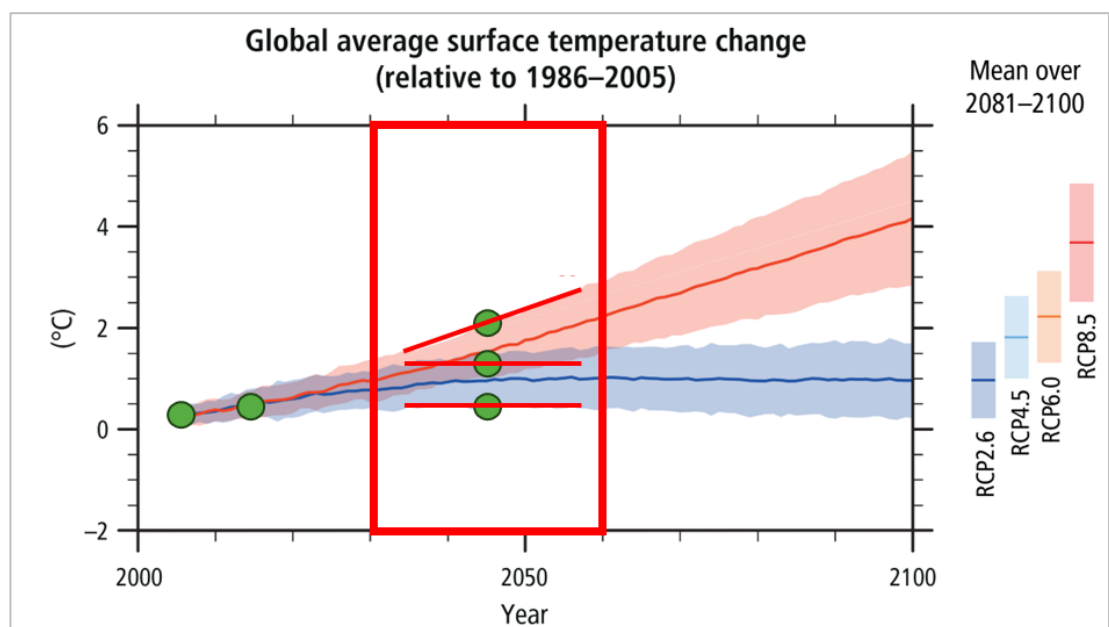
Abb. 6.2: Bandbreiten der globalen mittleren Temperaturänderung je nach RCP-Szenario, rot umrandet: die zu betrachtende nahe Zukunft, grüne Punkte: zu ermittelnde Grundwasserdargebote für den Ist-Zustand, das Trockenwetterdargebot und die drei RCP-Szenarien, verändert nach IPCC, 2014
