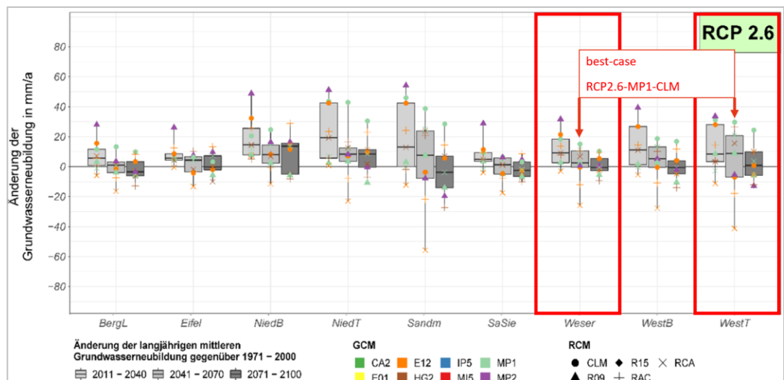
Abb. 6.4: Boxplots der Änderungssignale der langjährigen mittleren Grundwasserneubildung im RCP Teilensemble RCP2.6 („2 Grad Weg“) und den drei zukünftigen 30-Jahre-Perioden in den hydrogeologischen Großlandschaften. Fette Linien in den Boxen kennzeichnen die Mediane, die Boxen begrenzen den Interquartilsabstand, d. h. 50 % der Werte, aus HERMANN et al, 2021a
