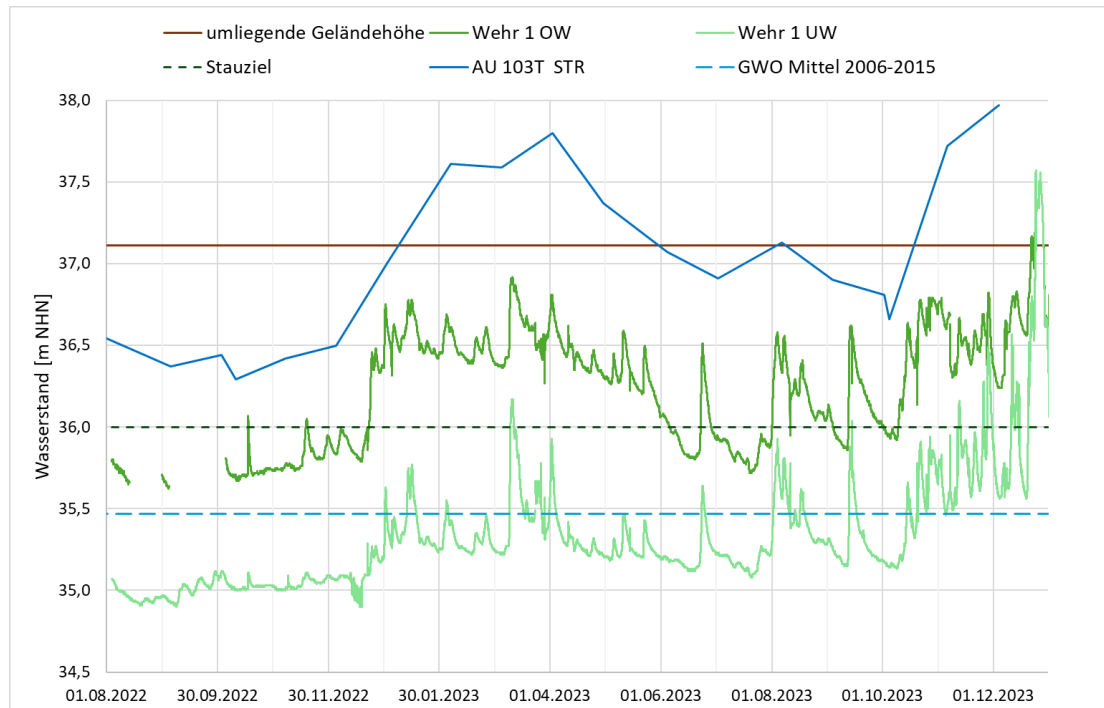
Abb. 6.9: Ganglinien des Oberflächenwasserstands im Ober- und Unterwasser von Stau 1 sowie der nächstgelegenen Grundwassermessstelle AU 103T Ströhen
