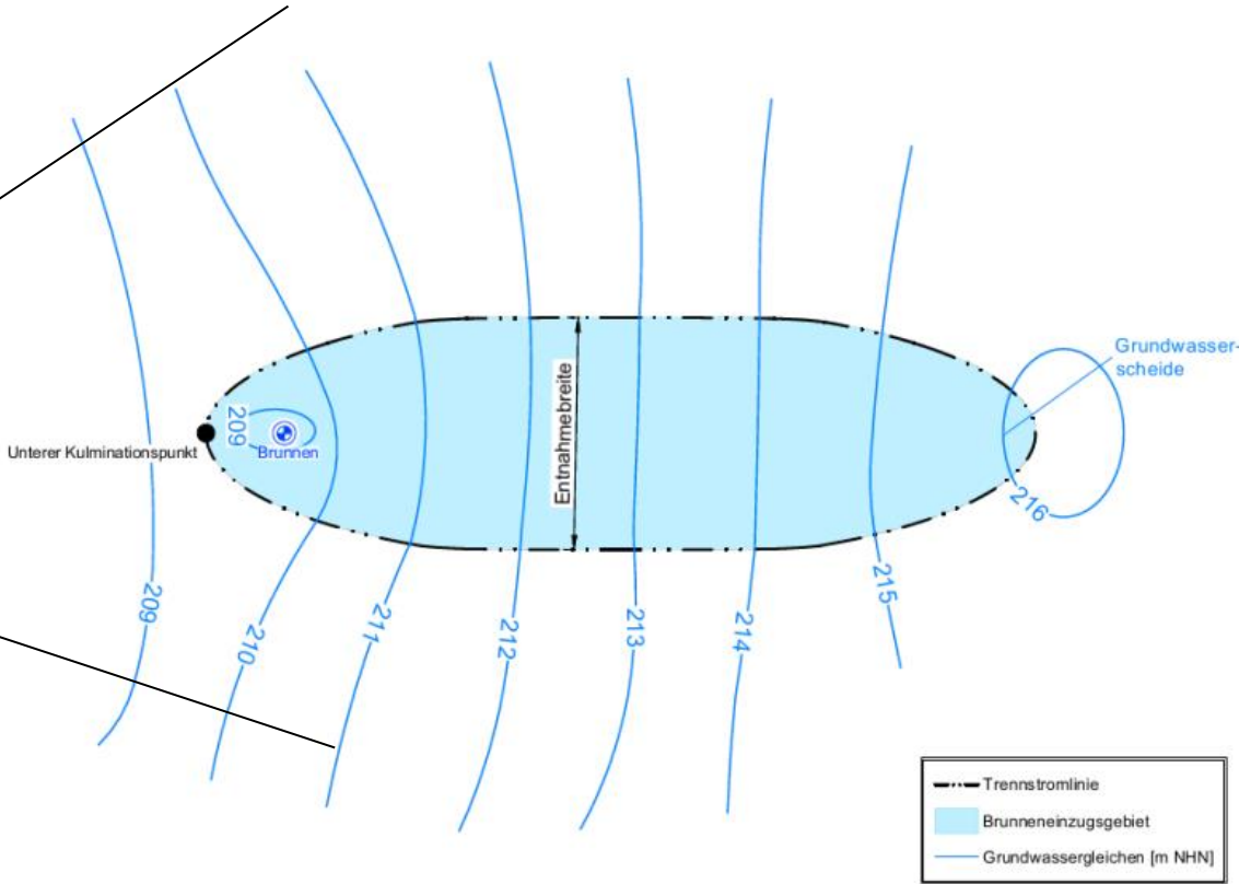
Unterirdisches Einzugsgebiet einer Grundwasserentnahme
