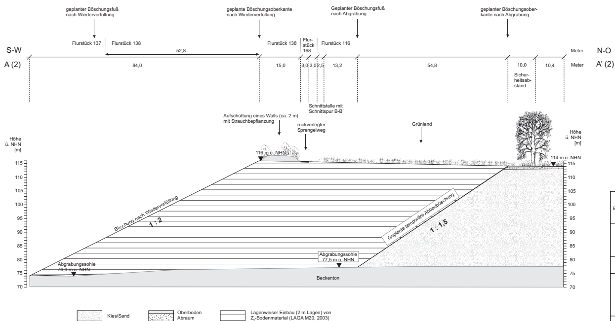
Schnitt A - A' durch die geplante Abgrabungserweiterung - nach Wiederverfüllung und Wegerückverlegung -
