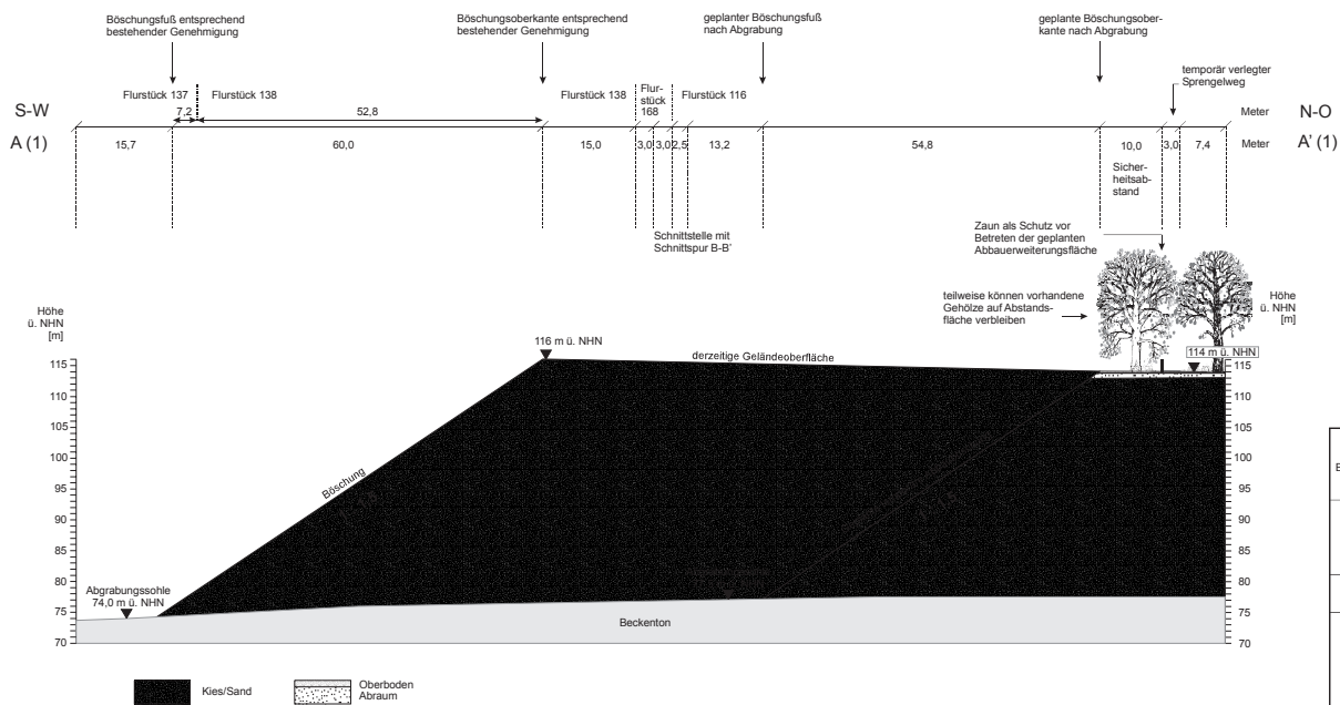
Schnitt A - A' (1) durch die geplante Abgrabungserweiterung - temporäre Wegeverlegung vor Beginn des Abbaus -
