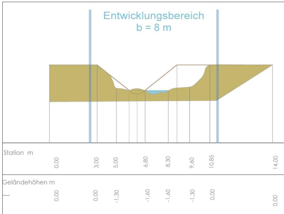
Abb. 4: Gestaltung des Westerbachs mit Sekundäraue
