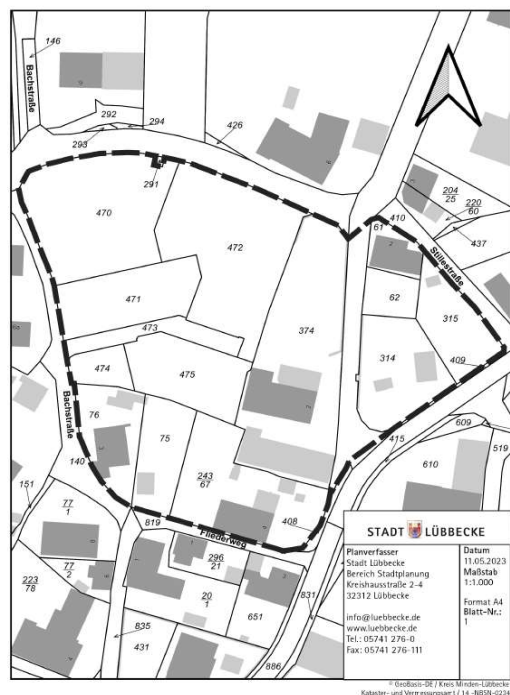
Geltungsbereich des Bebauungsplanes Nr. N 19 "Südlich Stillestraße / westlich Driffenstraße"
