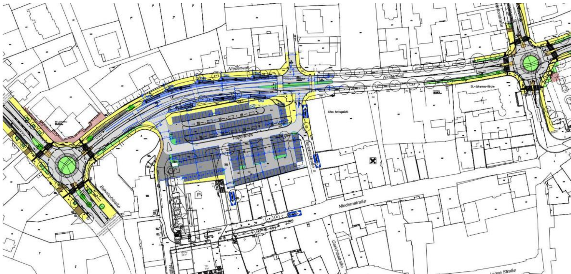
Abb.: Abbildung 2: Geplante Straßenstruktur der verkehrstechnischen Untersuchung
