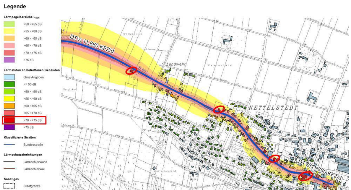
Abbildung 13: L_{den} der B 65 (Windmühlenfeld – Ravensberger Straße)
