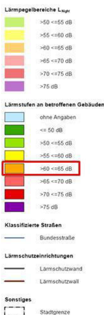
Abbildung 12: L_{Night} der B 65 (Mindener Straße – Nettelstedter Straße)
