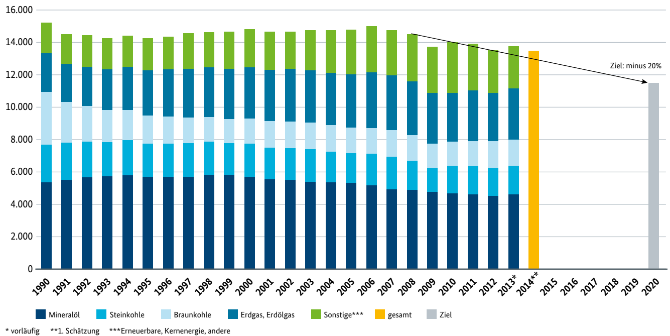
Abbildung 2: Entwicklung des Primärenergieverbrauchs nach Energieträgern bereinigte Werte in Petajoule (PJ)
